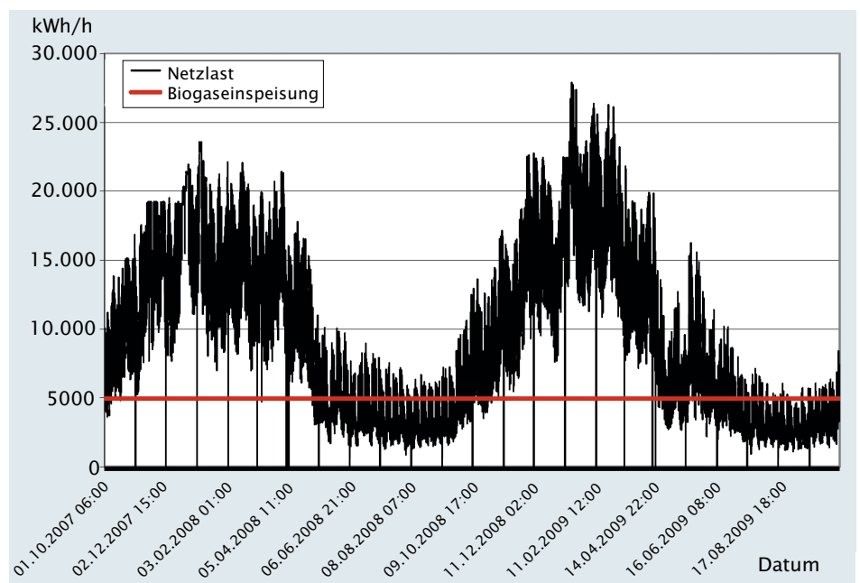
Beispielhafter Netzlastgang über zwei Jahre. In mehr als 29 % der Zeit („Sommersenke“) liegt die Netzlast unterhalb der konstanten Biogaseinspeisung von ca. 5000 kWh/h. Bild: BET
