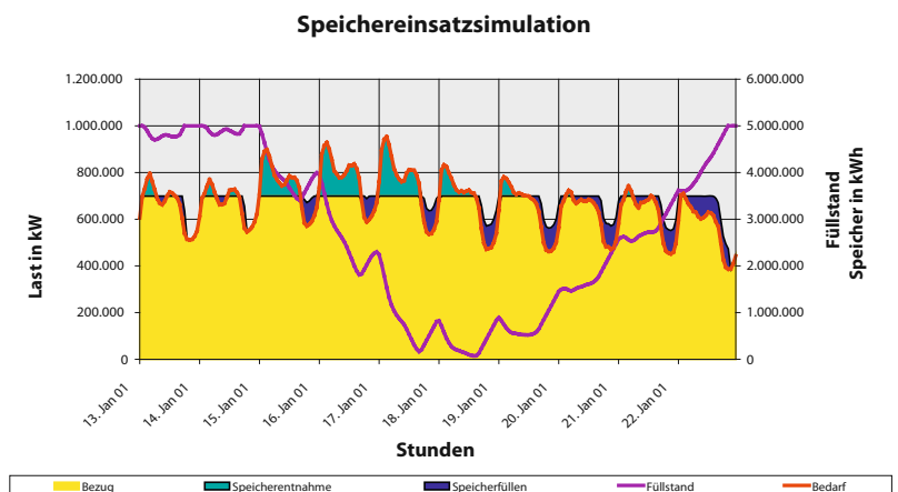
Bild 1. Beispiel Speichereinsatzsimulation.
